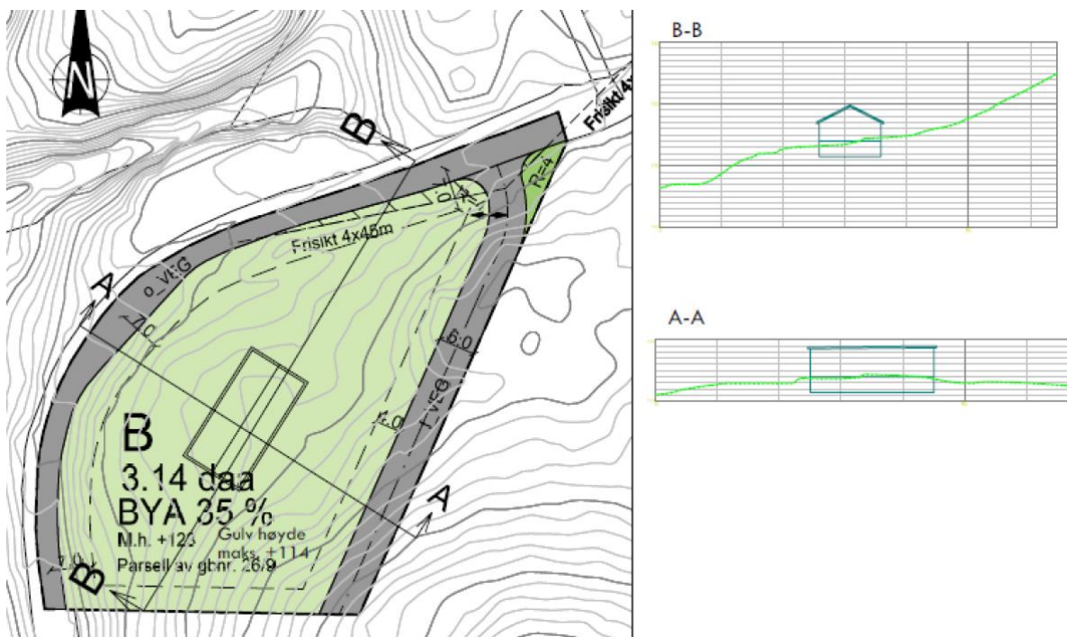
Figur 2. Snitt gjennom tomta. Som døme er det brukt ein bygning på 10 x 20 meter.
